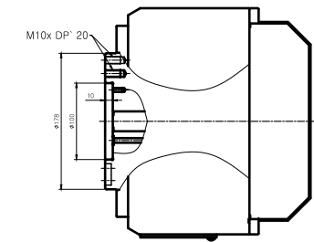
"회전축 단면도"
